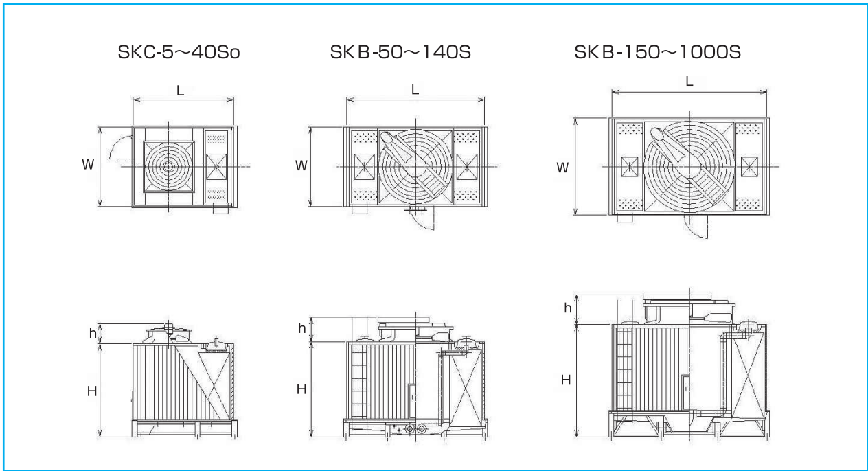
■ 騒音値表
