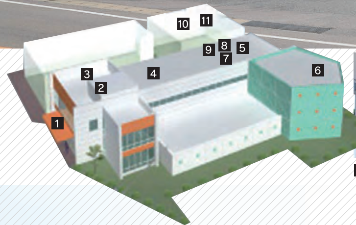
床面積 1,063m 2 建築面積 908m 2 気流試験エリア 126m 2 環境試験エリア 16m 2 残響室 300m 3 ダンパー試験室 146m 2
