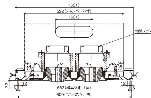
TAAC2正面図
