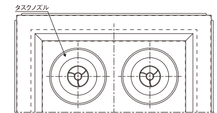
TAAC4正面図
