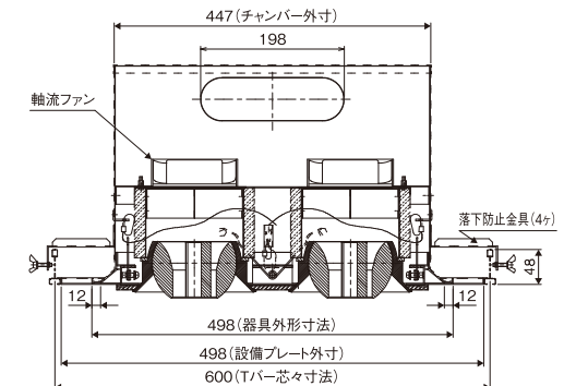
TAAC4側面図
