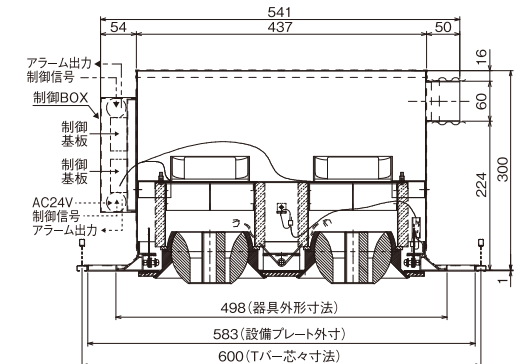
TAAC4側面図
