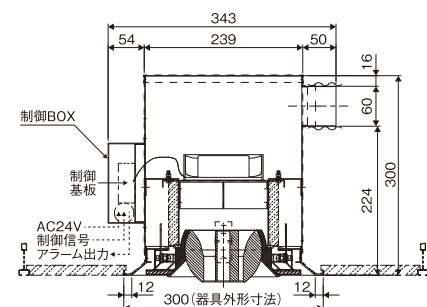
TAAC2側面図
