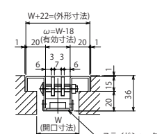
B-B断面図
