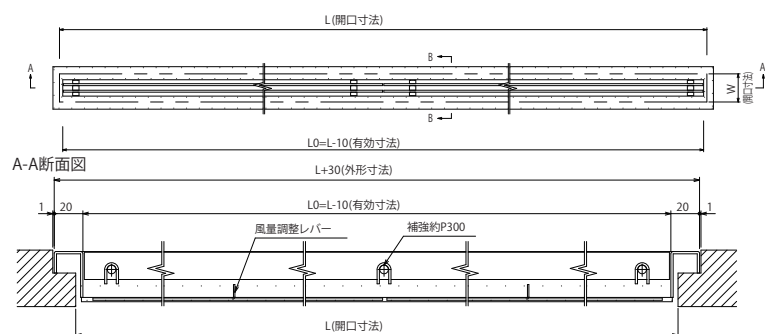
KFL-B(フラット額縁タイプ)
