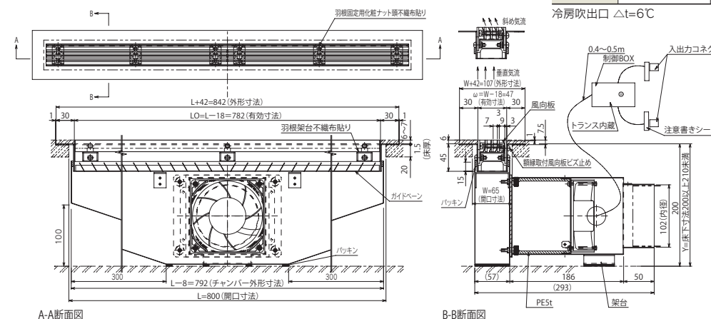
気流パターン① 【気流角度：垂直吹出】
