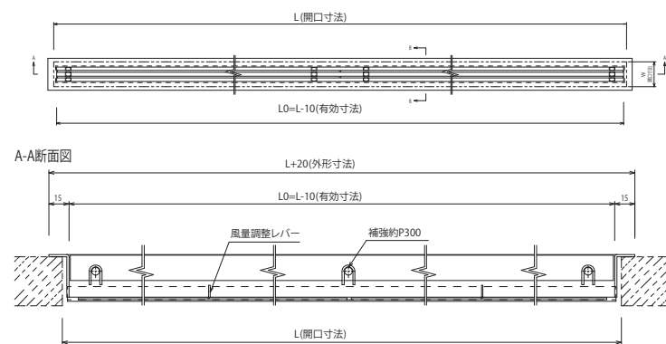
KFL-B(フラット額縁タイプ)
