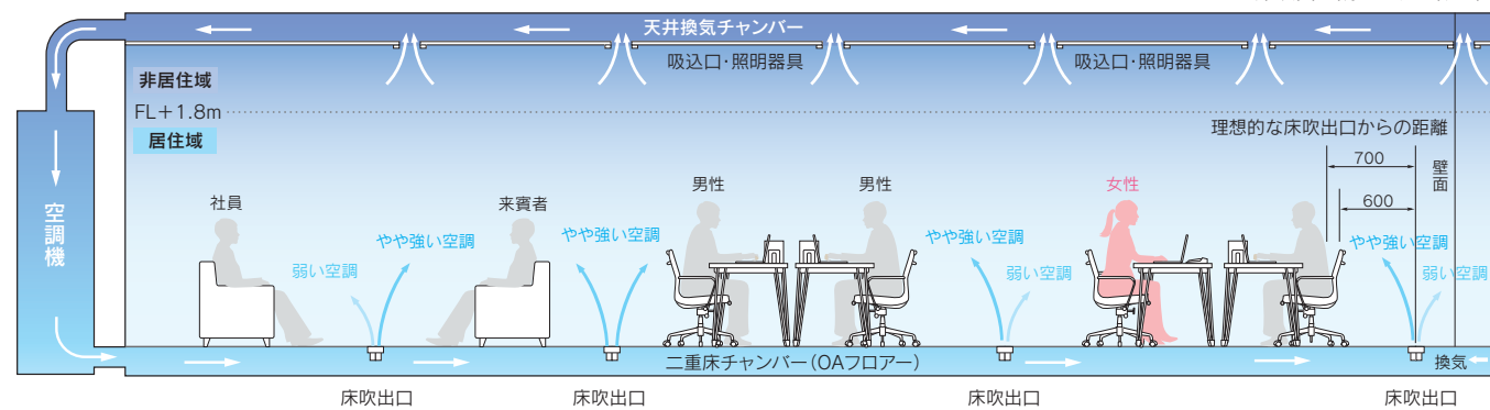
床吹出空調システム概念図
