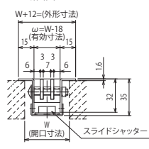
B-B断面図
