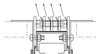
気流パターン③ 【気流角度：14°】
