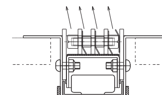
気流パターン④ 【気流角度：8°】
