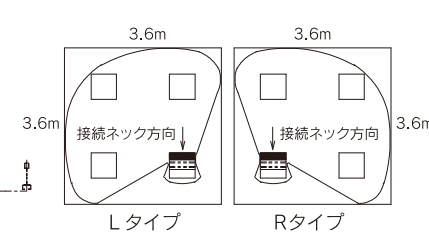
気流パターン (平面図)
