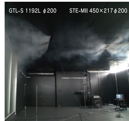
GTL-S 1192L インテリア・ベリ側気流(冷房)
