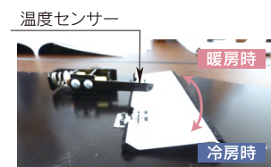
可動偏向板拡大写真
