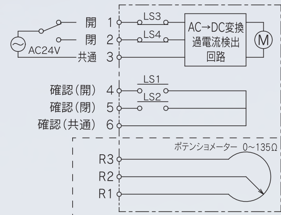
KGM-3型内部回路図
