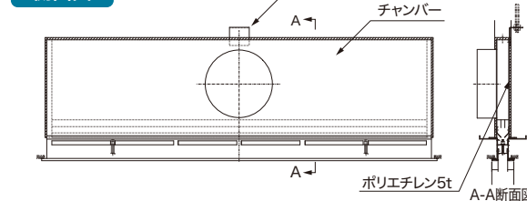
側面図
