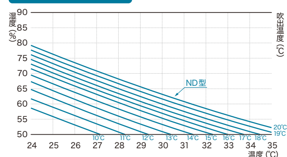
結露限界曲線 (#4~14)
