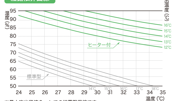
結露限界曲線
