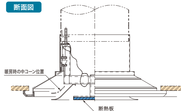
断面図
