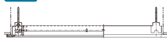
側面図
