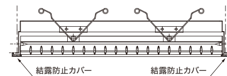
断面図
