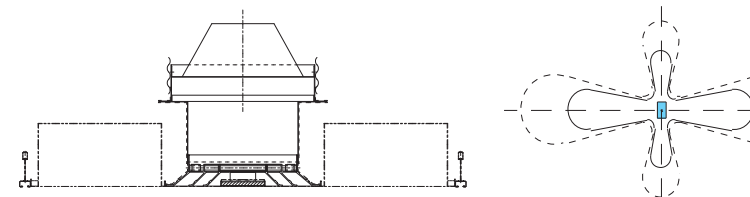
断面図
