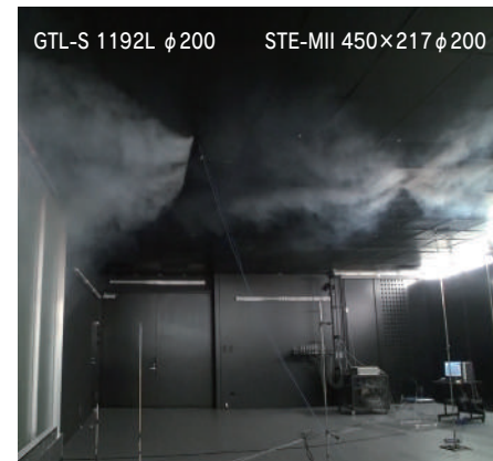
GTL-STE-MII インテリア・ペリメータークロス(冷房) 風量：300CMH (STE-MII) 200CMH (GTL) 温度：温度差 \Delta t=13^{\circ}\text{C}
