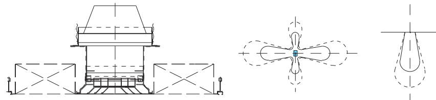
断面図
