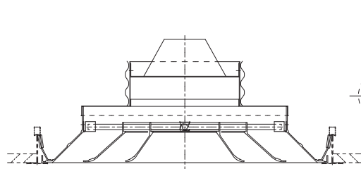
断面図
