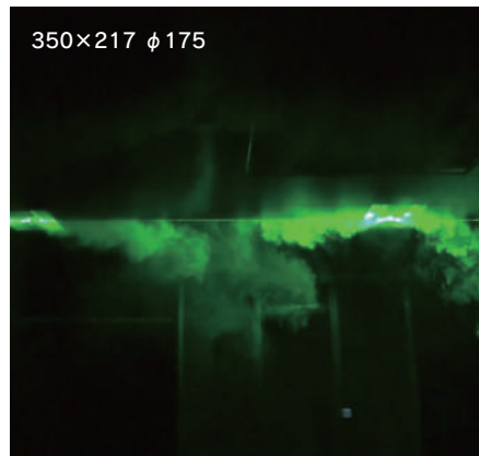
STE-MII 干渉(冷房) 風量：250CMH×2台 温度：温度差 \Delta t=13^{\circ}\text{C}
