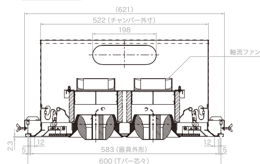
側面図
