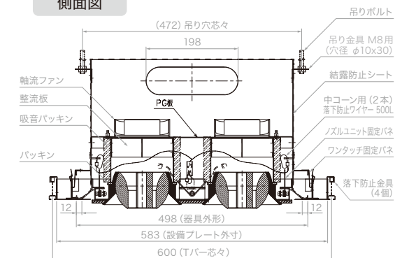
側面図
